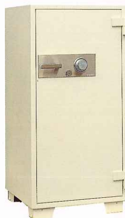
No.500 ②TS ¥248,000 外寸法/610W×640D×1,250H 内寸法/450W×444D×1,010H 内容積/202 Q 重量/260kg 附属品/棚板3枚
